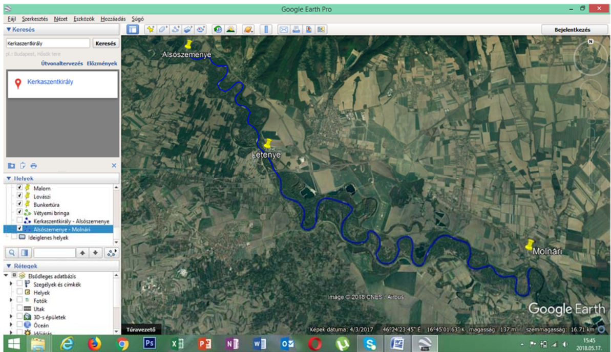
Útvonal Alsószerényétől Molnárrig (Forrás Google Earth)
